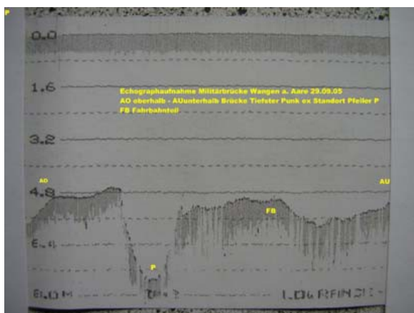
Flussbettprofil mit Echograph
